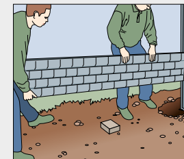
Erste Motivplatte nach gewünschter Flucht in die Nut setzen und mit dem Acryl verkleben. Ende der Platte mit einem Pflasterstein als stabile Auflage unterlegen und Motivplatte in Waage setzen.
