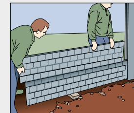
Motivplatten entsprechend der passenden Seite in die Pfostennut einsetzen und weiter verkleben. (Bei dem Motiv Nostalgie Z-Versatz beachten, bei Klassik-Stein A und B Seite im Wechsel einsetzen)
